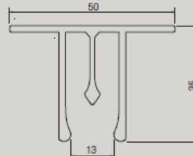
FUM-D01 ＜二重レール＞
