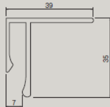
FUM-C01 ＜単独レール＞
